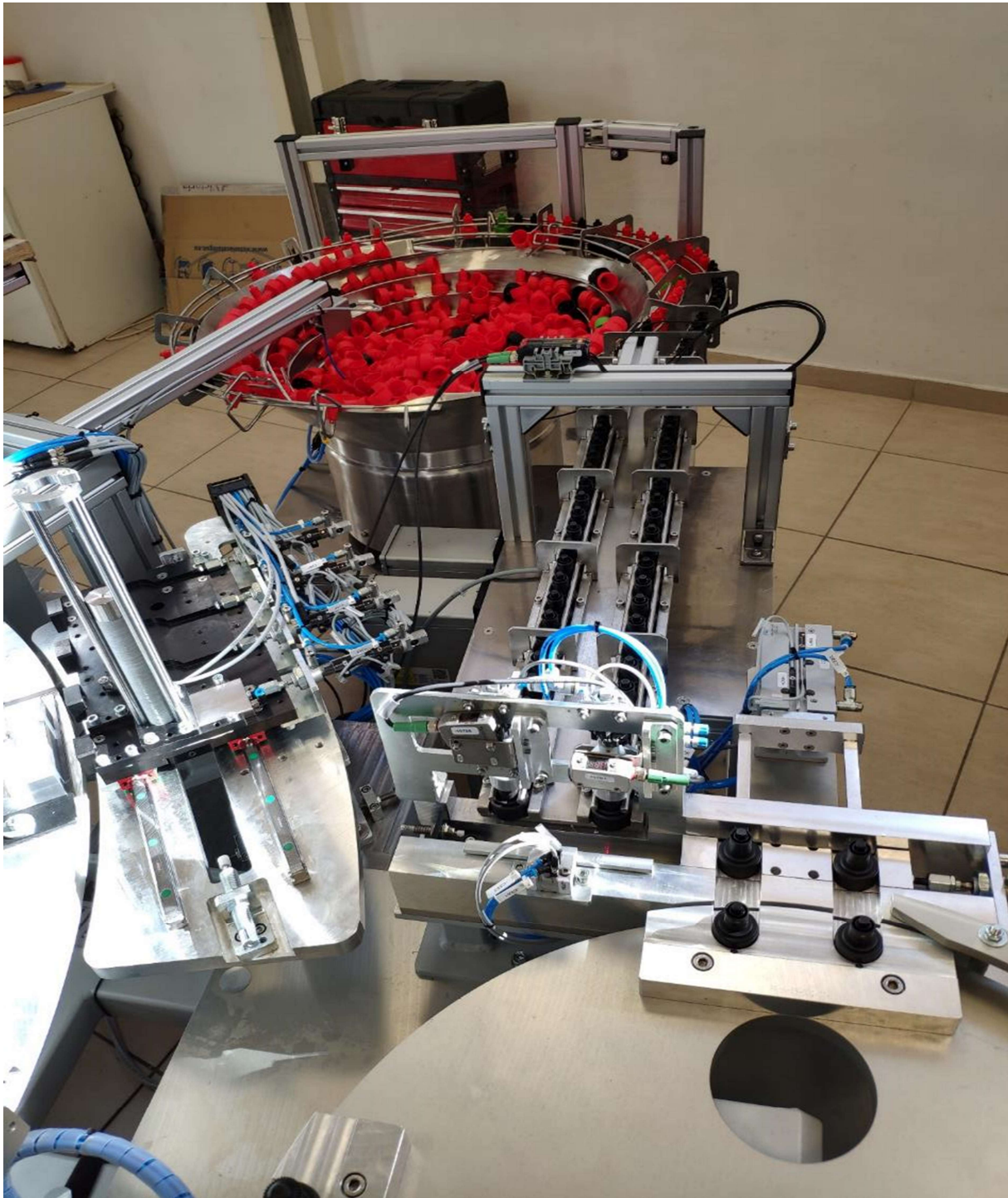
7. kép Kupak rezgődob
