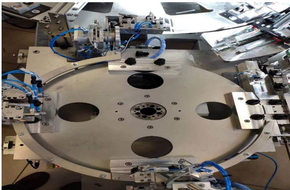
5. kép Kupak összeszerelő asztal
