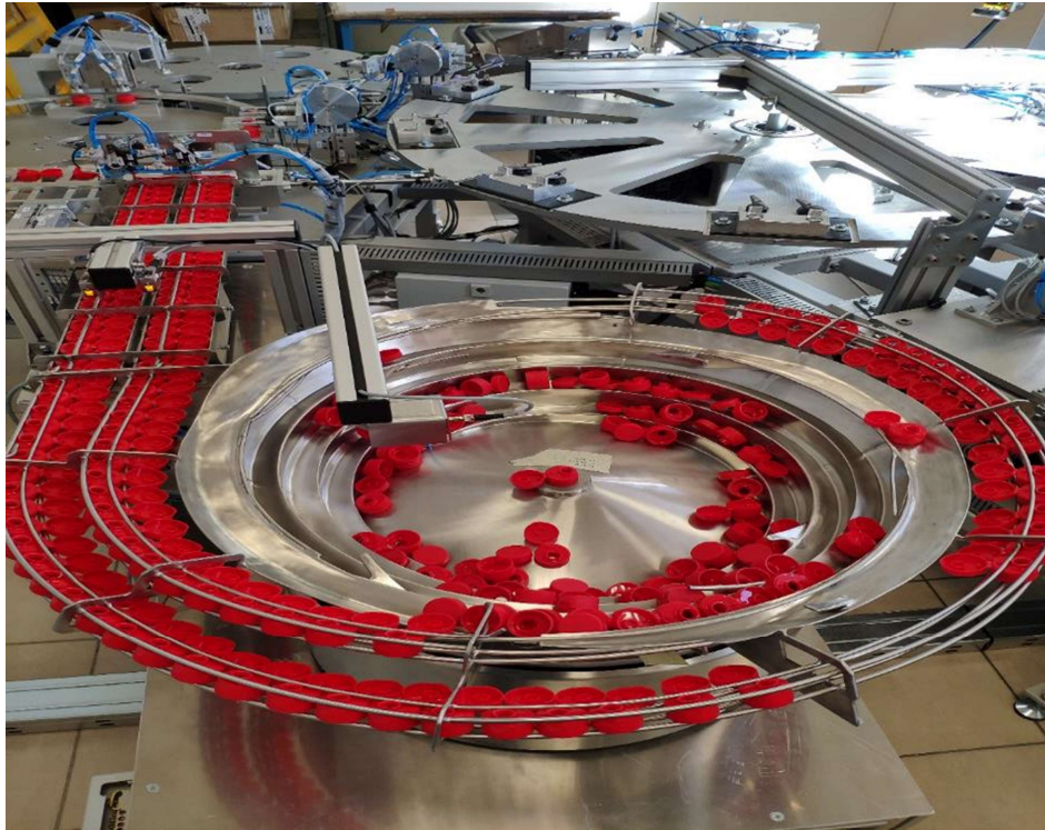
4. kép Rázó- és szortírozó dob
